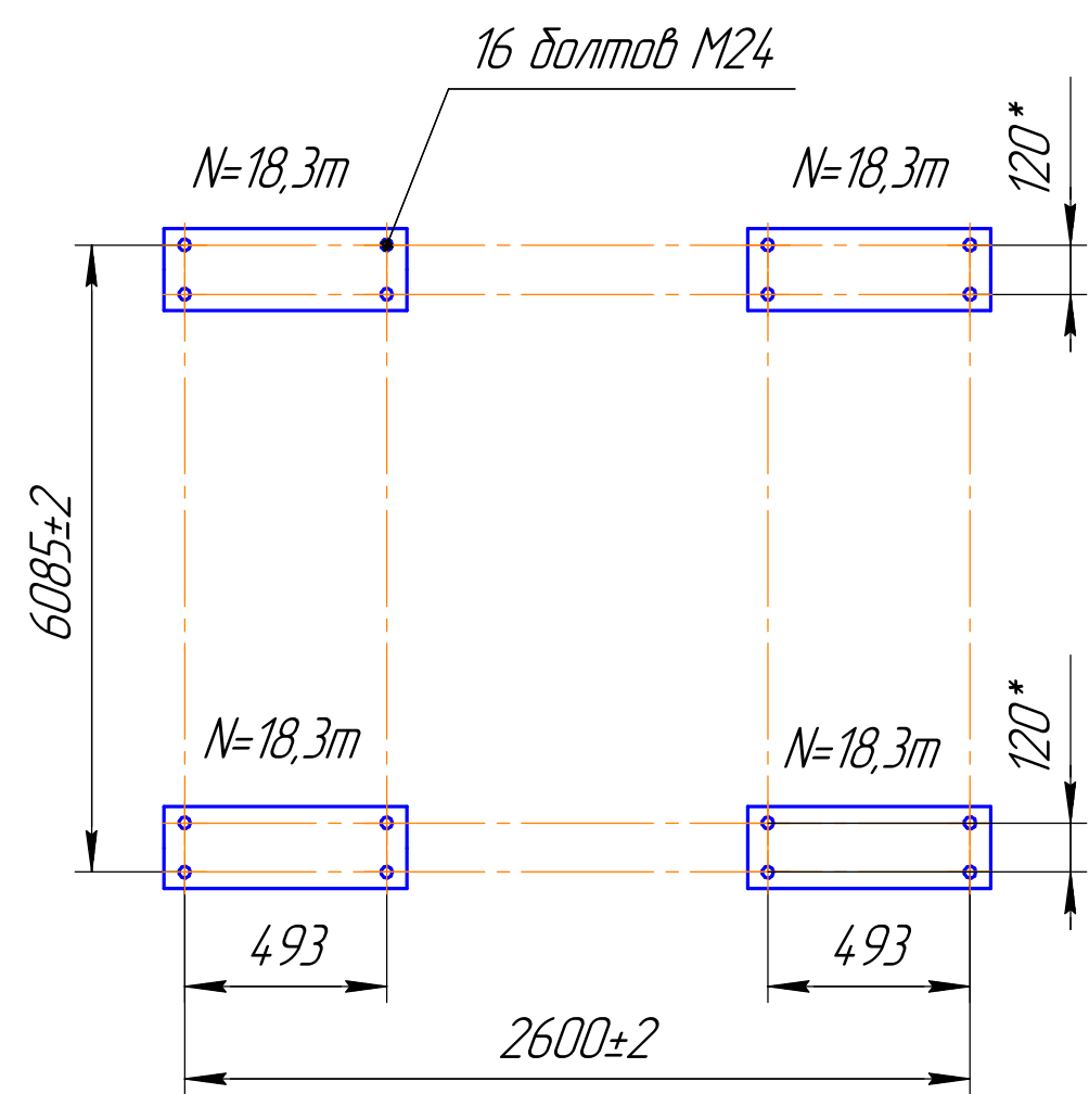
План расположения болтов
