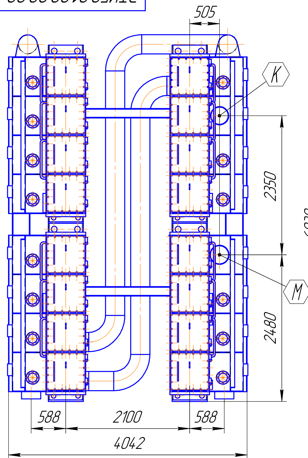
План расположения болтов
